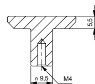
A-A (1 : 1)
