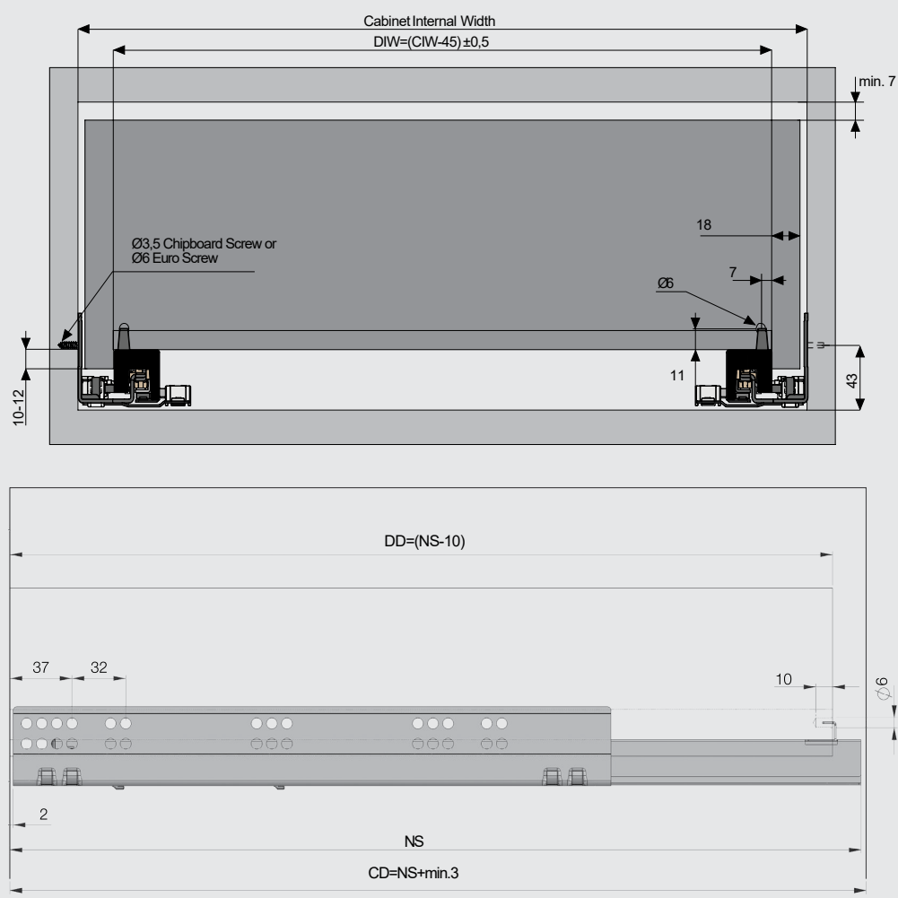
POZICIJE VIJAKA
